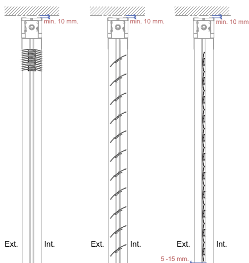
Sección vertical
