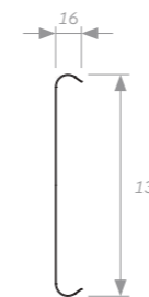
Sección lama (cotas en mm)
